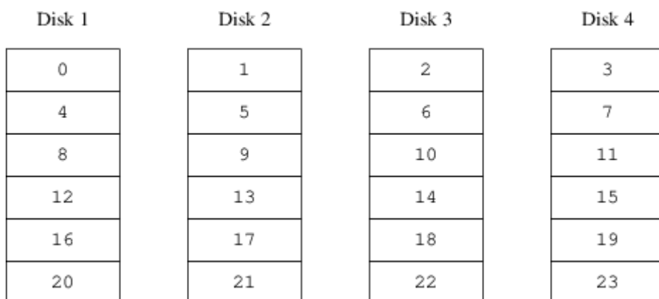
Ábra 60. A csíkozott szervezési mód
