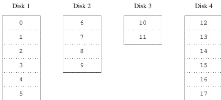
Ábra 59. Az összefűzött szervezési mód
