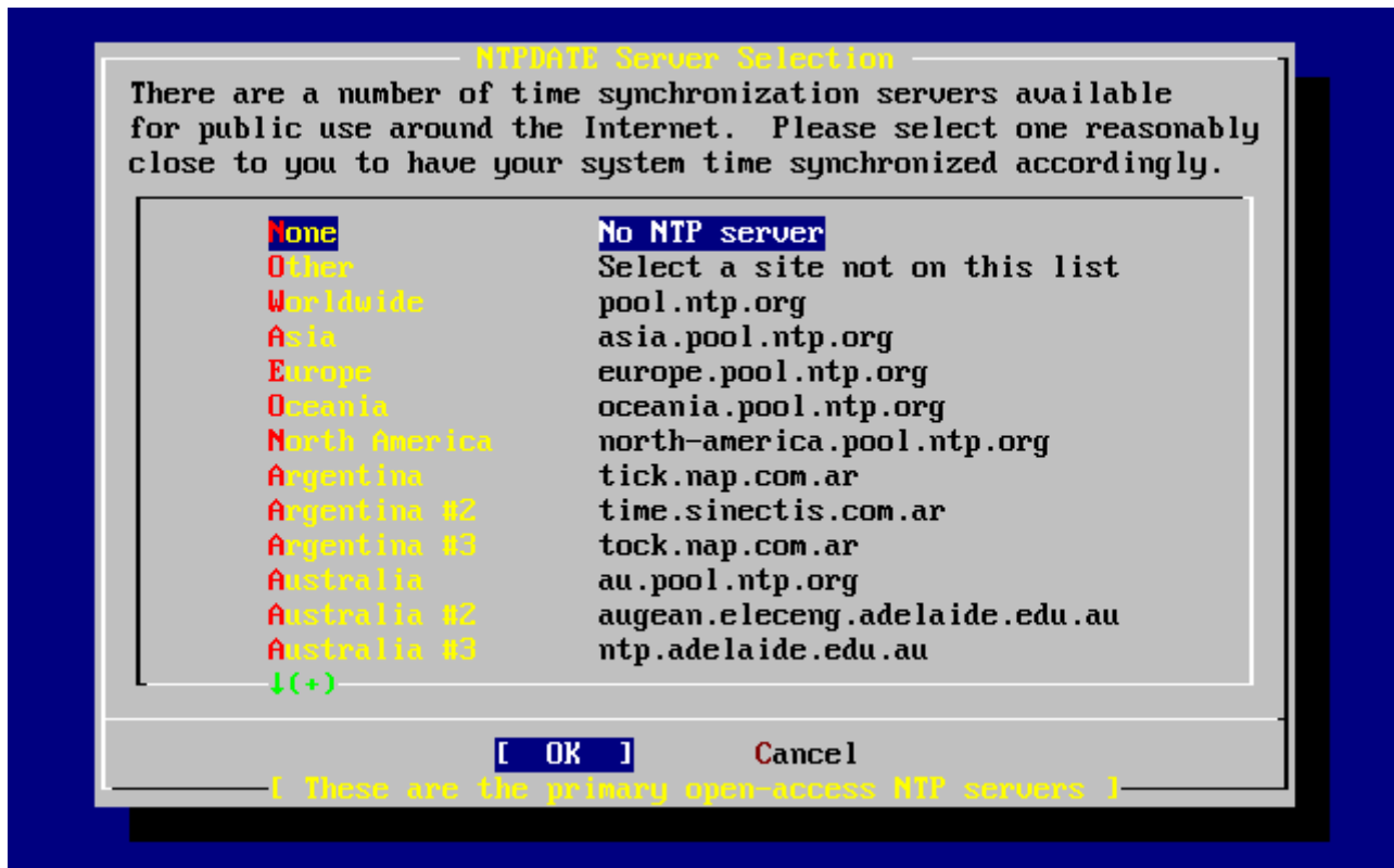
Рисунок 56. Настройка Ntpdate
